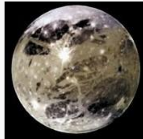
Ganymede
