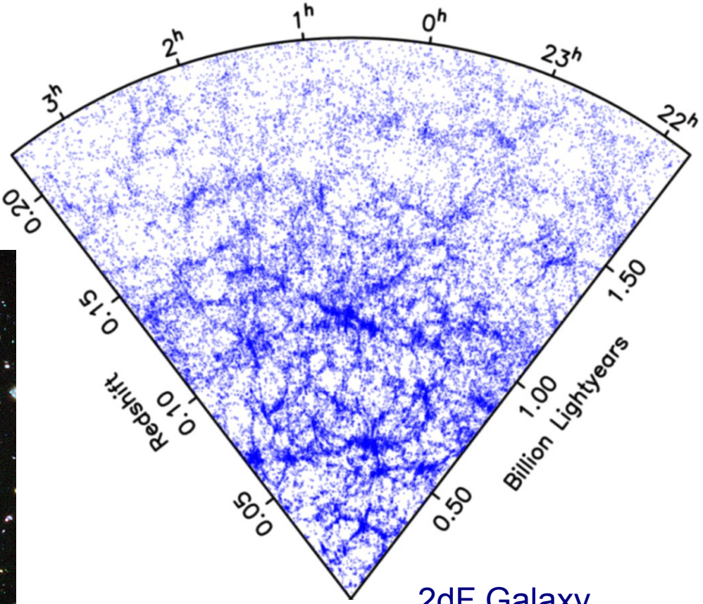
2dF Galaxy Redshift Survey
