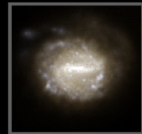
disk galaxies
