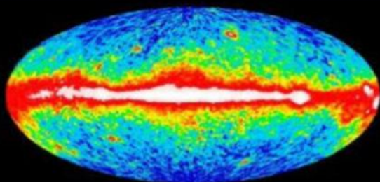
Gamma-Ray >100\text{MeV} (CGRO, NASA)
