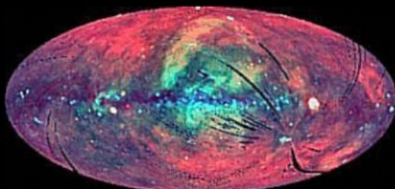
X-Ray 0.25, 0.75, 1.5\text{ keV} (S. Digel et.al. GSFC, ROSAT, NASA)
