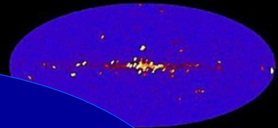
X-ray 0.25, 0.75, 1.5 keV (AXE-1, NASA)
