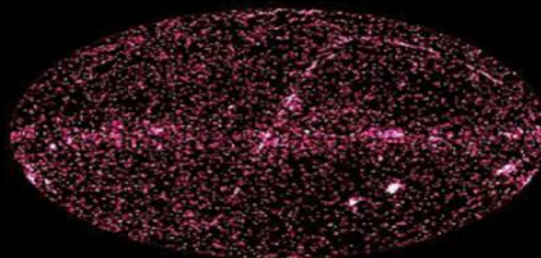
Ultraviolet (J. Bonnell et.al.(GSFC), NASA)
